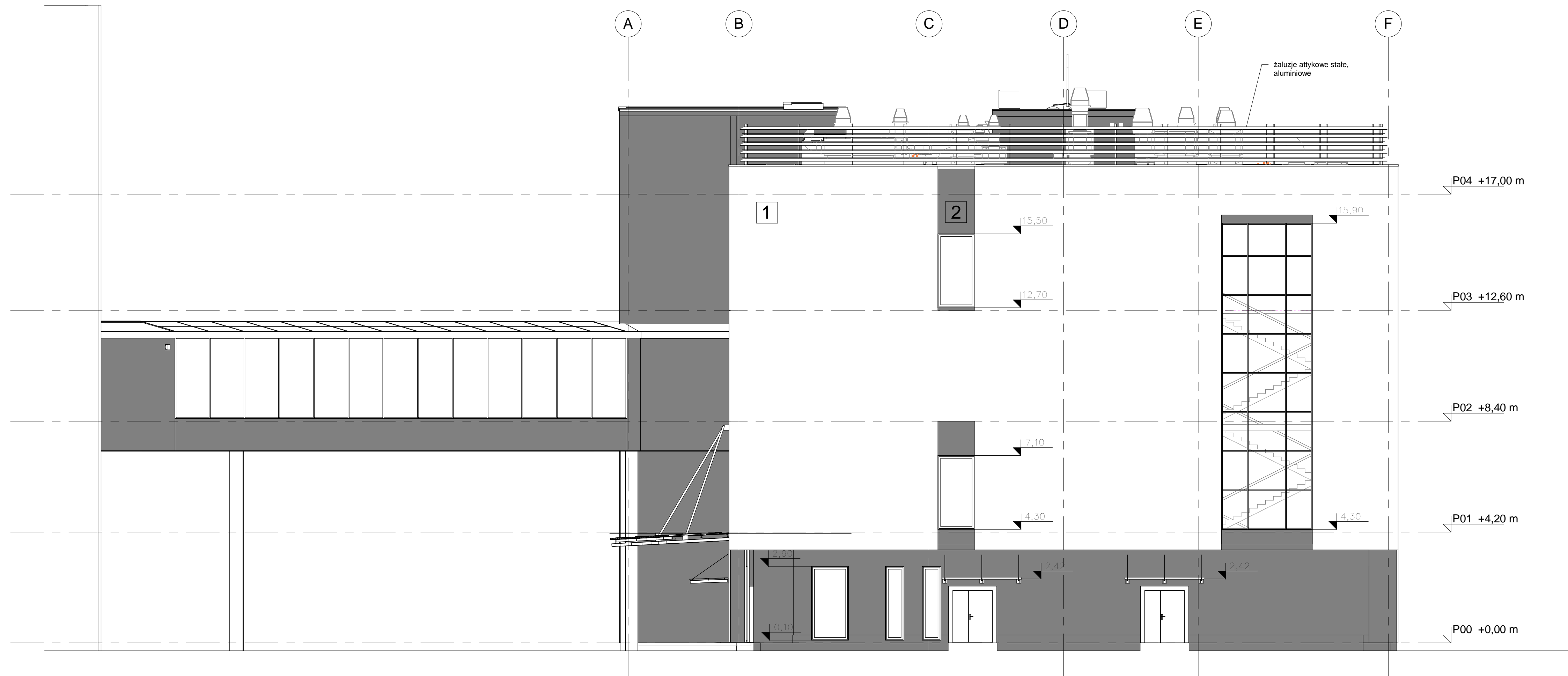
ELEWACJA WSCHODNIA
