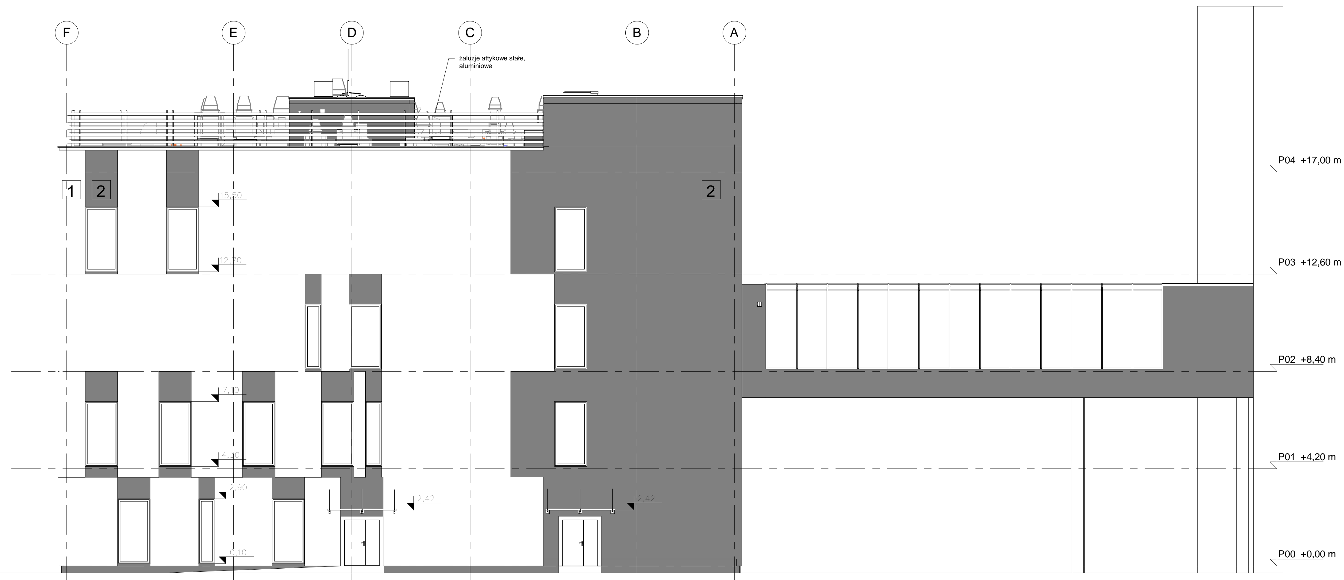
ELEWACJA ZACHODNIA
